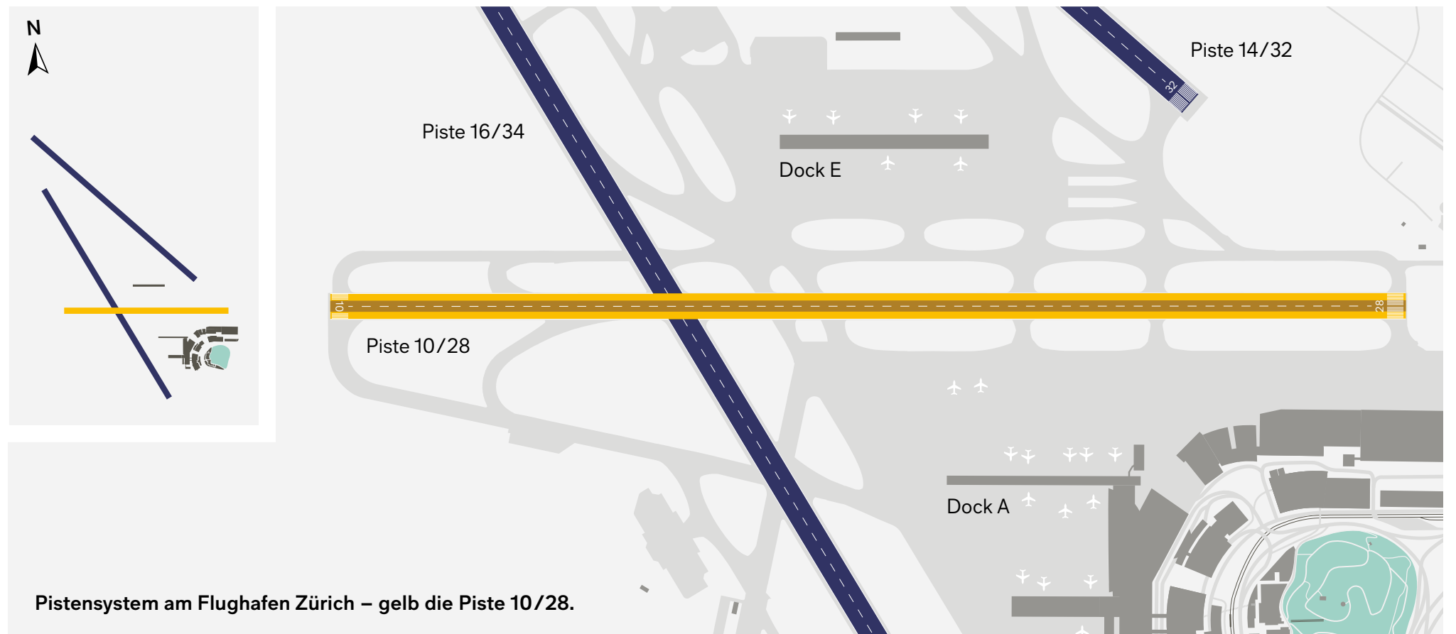
Bei der Pistensanierung wird der 22.8 m breite Mittelstreifen der Piste 10/28 saniert.
